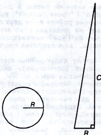
Архімедава сувязь круг-трохвугольнік
