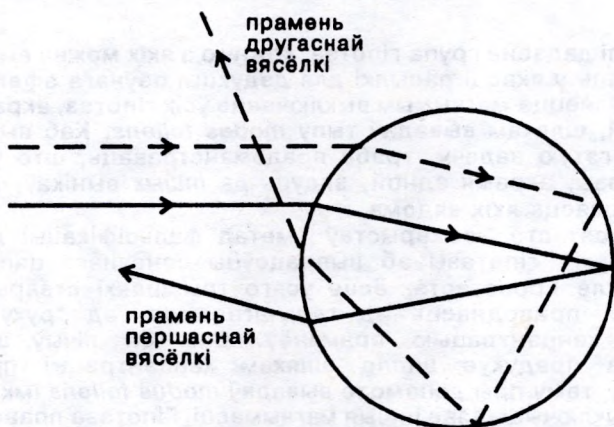
Мадэль дажджынкі Тэадарыка
