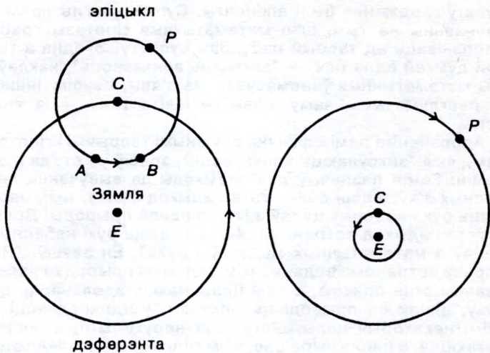
Эпіцыклічна-дэферэнтная мадэль
