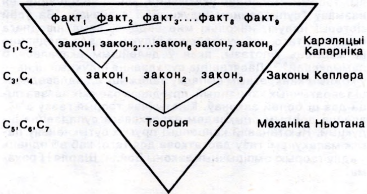
Індукцыйная табліца Уэвэла.
