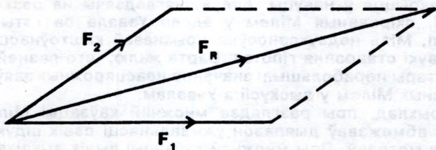
Паралелаграм сіл
