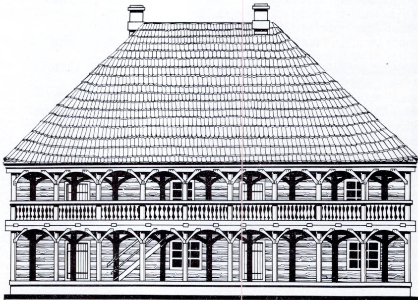
67. Лямус у брыгіцкім кляштары ў Гродна. Фасад. Канец XVII ст.
