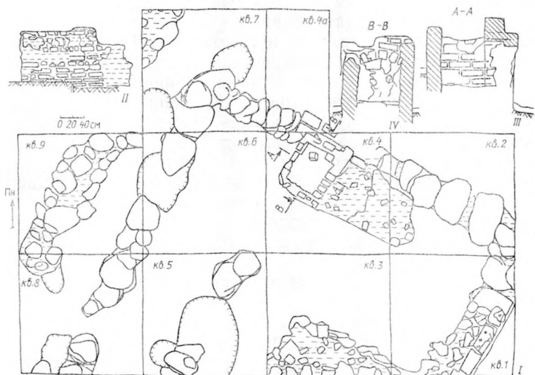
6. План раскопу рэшткаў будынка 2-й паловы 17 ст. з кафлянай печкай (раскоп 3—1984 г.). I—план раскопу 3; II—сістэма муруўкі тулава кафлянай печы; III—разрэз А—А; IV—разрэз В—В
