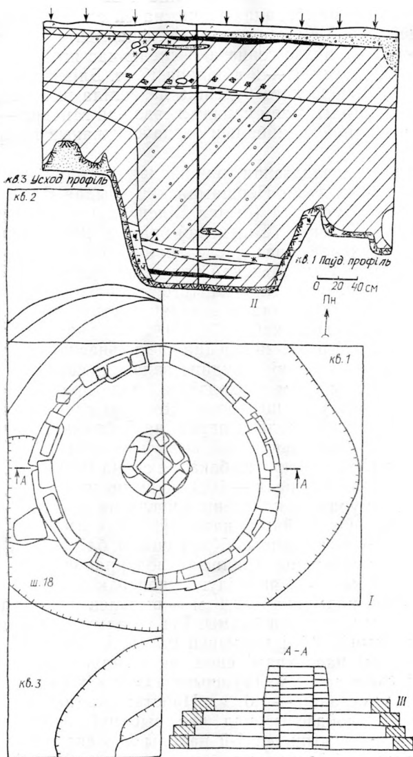
7. Раскопки рэштак горна 2-й паловы 17 ст. для абпалу керамікі (раскоп 2 — 1983 г.). I — план раскопу 2; II — профілі раскопу 2; III — разрэз горна
