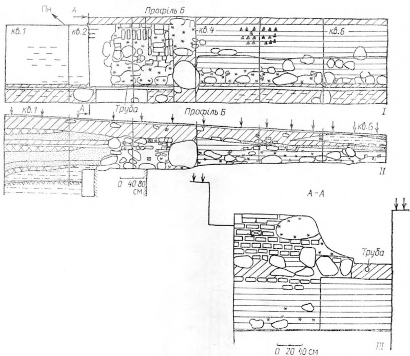
8. Раскопкі рэшткаў Віленскай брамы (траншэя 3 — 1988 г.). I — план траншэі; II — профіль Б; III — разрез А—А
