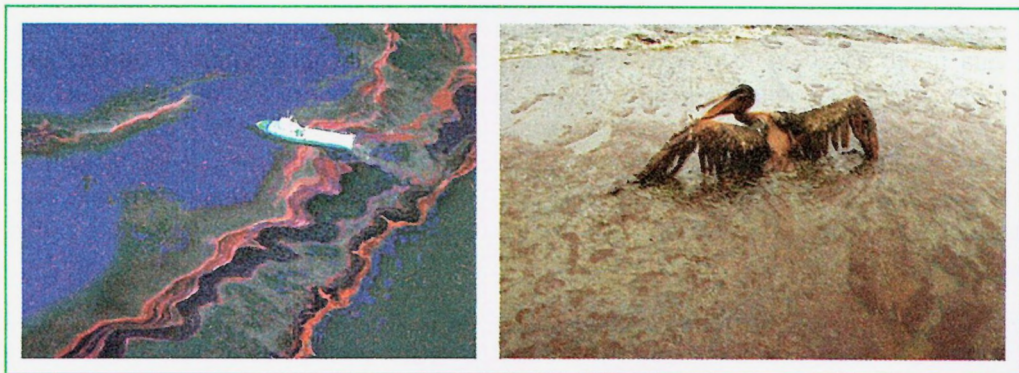
Мал. 100. Наступствы аварыі ў Мексіканскім заліве
