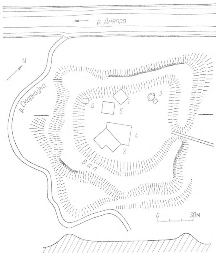
План Копыскага замчышча
