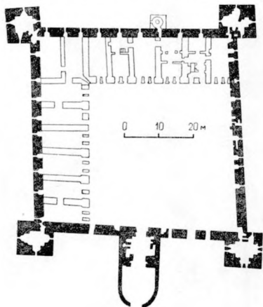
План замка (паводле А. Я. Міцяніна і аўтара)
