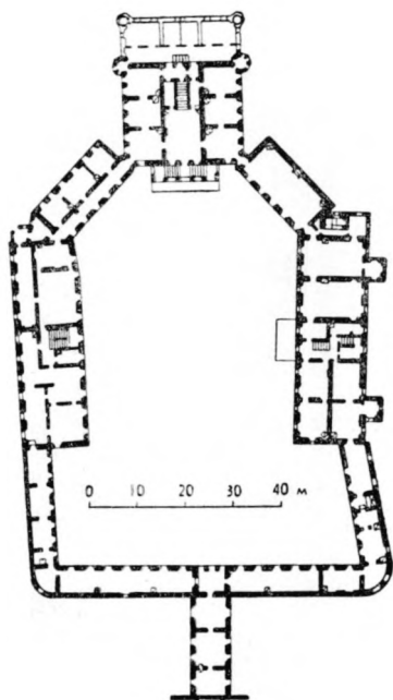
План першага паверха Нясвіжскага замка
