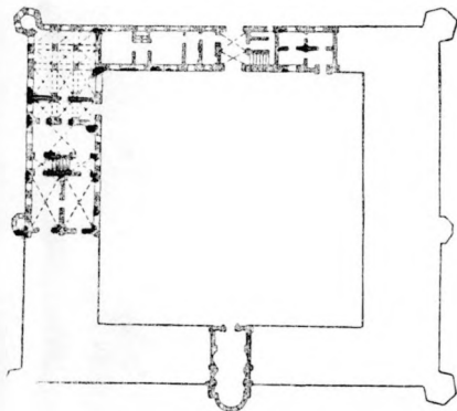
План першага паверха Гальшанскага замка
