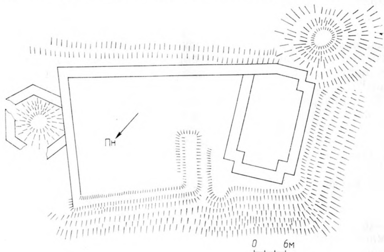
План Іказненскага замка
