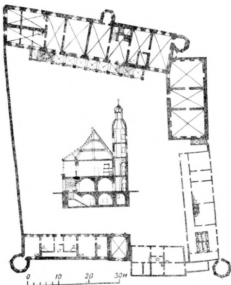
Быхаўскі замак. План першага паверха
