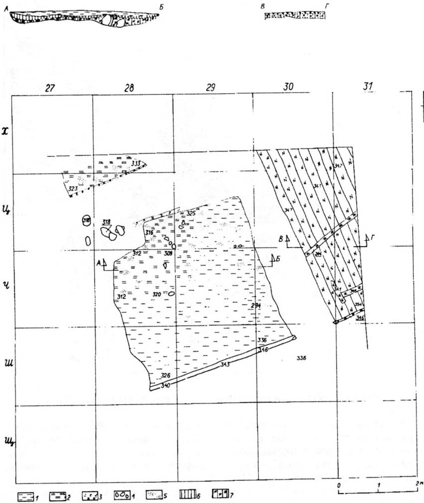
Мал. 124. Замкавая гара. Раскоп 3. Пабудова 29. Вымастка з гліны. 1 — неабпаленая гліна, 2 — абпаленая гліна, 3 — сатлелыя дошкі, 4 — камяні, 5 — пясок, 6 — гумус, 7 — гумус з шчэпамі.
