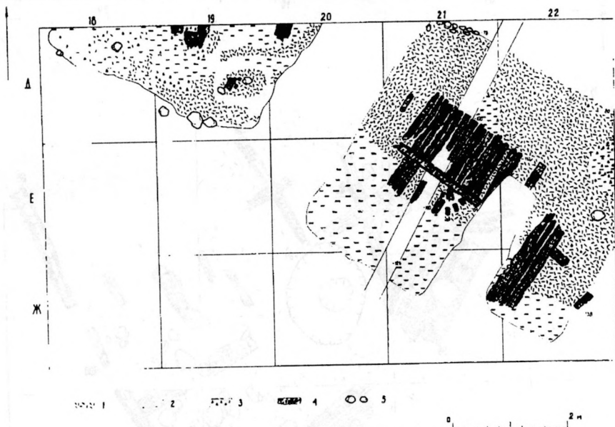
Мал. 113. Замкавая гара. Раскоп 1. Пабудова 9а, план. 1 — вугаль, 2 — неабпаленая гліна, 3 — зала, 4 — гарэлае дрэва, 5 — камяні.
