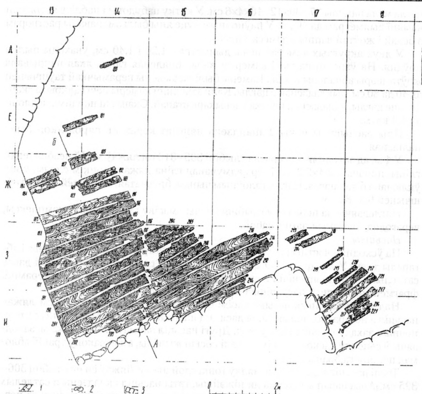
Мал. 119. Замкавая гара. Раскоп 1. Насыціл III, план. 1 — сатлелае дрэва, 2 — камяні, 3 — граніца пабудовы XIV ст.
