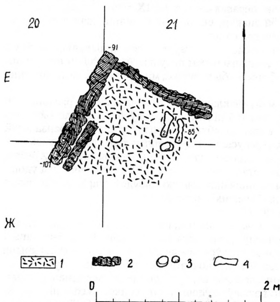
Мал. 115. Замкавая гара. Раскоп 1. Пабудова 6, план. 1 — вугаль, 2 — гарэлае дрэва, 3 — камяні, 4 — тачыльны камень.
