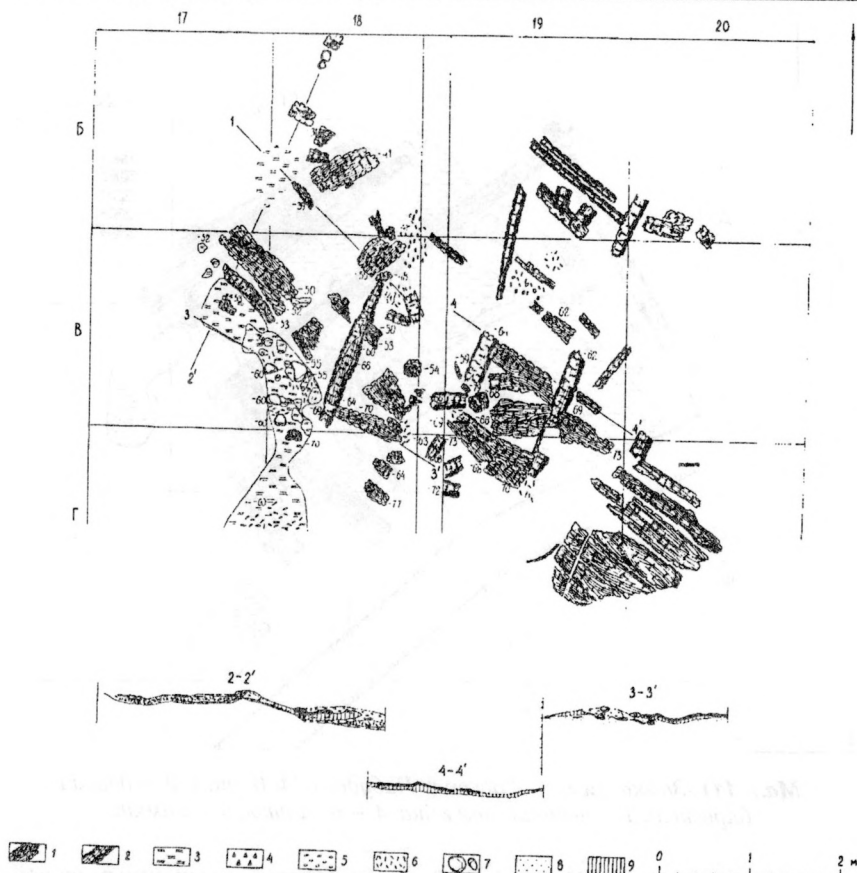
Мал. 112. Замкавая гара. Раскоп 1. Пабудова 15, план. 1 — гарэлае дрэва, 2 — сатленае дрэва, 3 — неабпаленая гліна, 4 — зала, 5 — тлен дрэва, 6 — вугаль, 7 — камяні, 8 — пясок, 9 — гумус.
