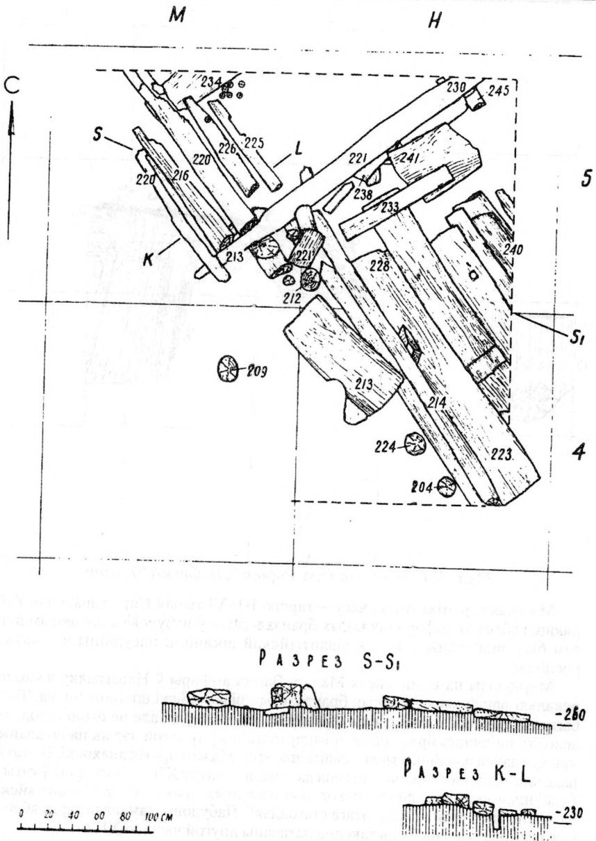
Мал. 122. Замкавая гара. Раскоп 2. 1 — пабудова 4, 2 — пабудова 3. Пляны.
