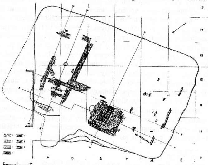
Мал. 15. Малы Замак. Пабудова 5. План: 1 - неабпаленая гліна, 2 - абпаленая гліна, 3 - вапнавы раствор, 4 - гарэлае дрэва, 5 - сатлейшая падлога, 6 - камяні, 7 - цэгла.
