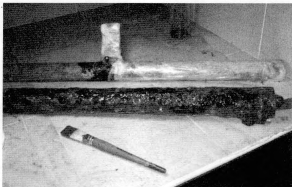
Іл. 9. Гакаўніцы (КП 5359 і КП 5360) пранітаныя пераўтваральнікамі іржы “Крышталь-Р” і “Анкор-1”.
