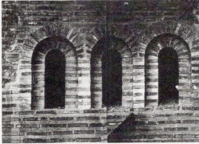
Іл. 19. Муроўка са схаваным радам. Царква Міхаіла Арханёла ў Смаленску.
