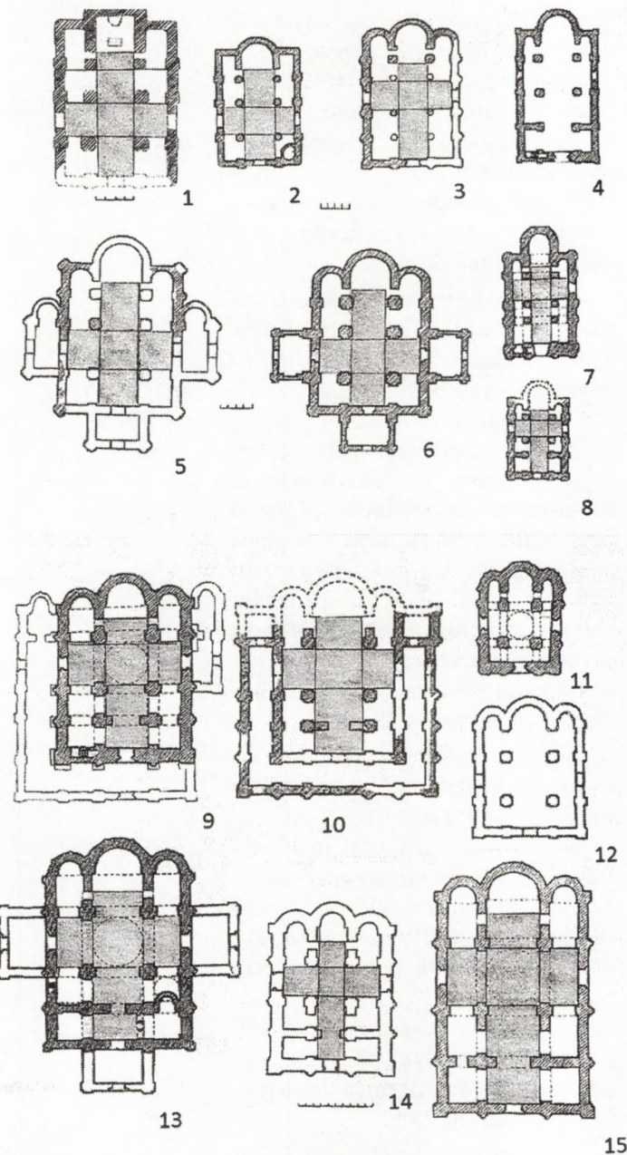
Іл. 33. Пляны крыжова-купальных храмаў XII ст.: 1 — Прачысценская царква, 2 — Ніжняя царква, 3 — Каложская царква (Гародня); 4 — Дабравешчанская царква (Віцебск); 5 — царква на дзядзінцы, 6 — вялікі сабор Бельчыцкага манастыра, 7 — Спасаўская царква Спасаўскага манастыра, 8 — Барысаглебская царква Бельчыцкага манастыра (Полацк); 9 — Барысаглебскі сабор, 10 — Дабравешчанская царква, 11 — Пятніцкая царква, 12 — Міхайлаўская царква, 13 — Успенскі сабор Ялецкага манастыра (Чарнігаў); 14 — Старая кафедра, 15 — Успенскі сабор (Уладзімір-Валынскі). Паводле П. Рапапорта.
